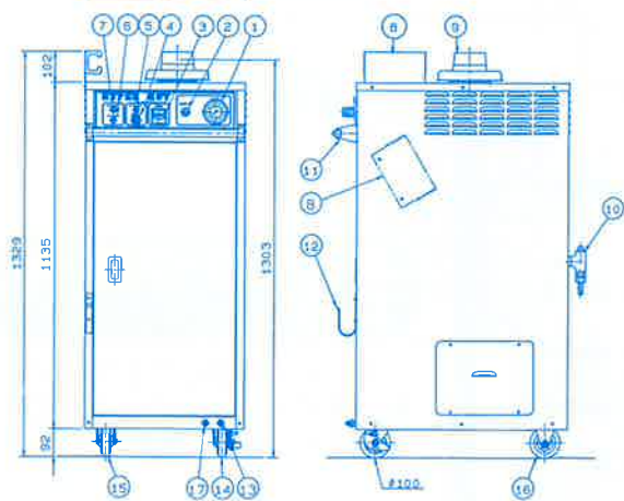
●寸法図
