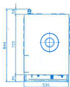
●寸法図
