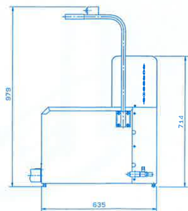
●寸法図
