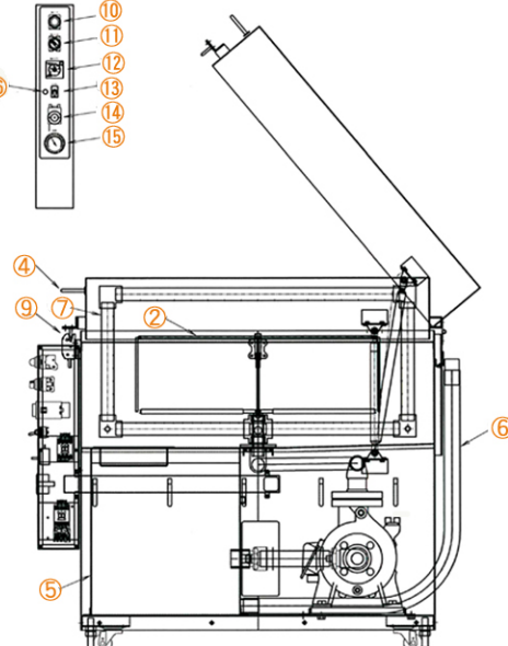
操作部詳細
